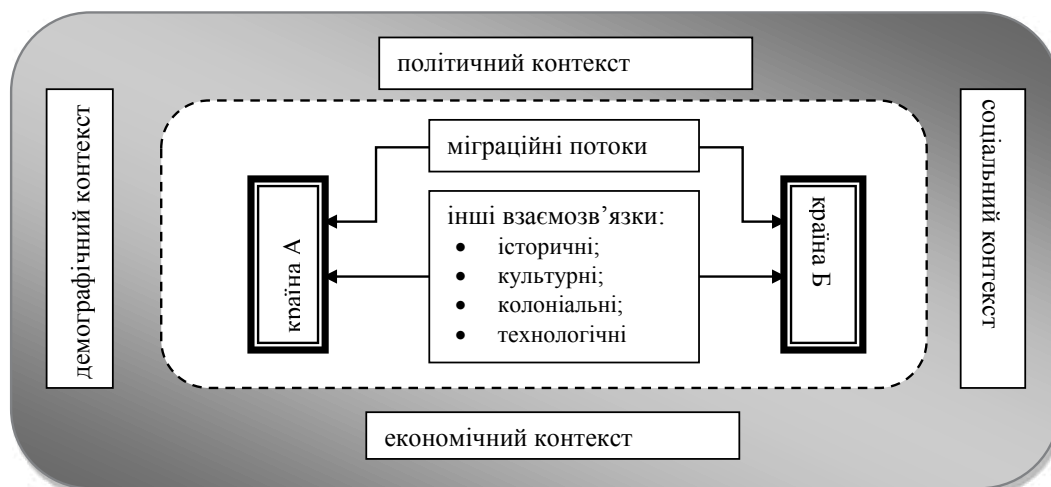
Рис. 2. Графічне зображення міграційної системи на макрорівні
