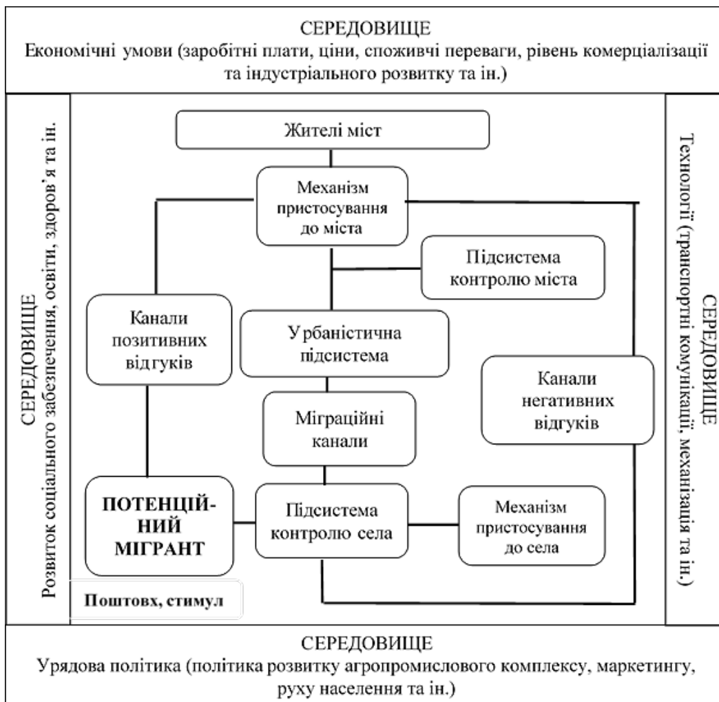
Рис. 1. Схематичне зображення урбаністичної міграційної системи за А. Мабогундже [12, с. 3]
